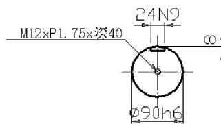
出力軸
